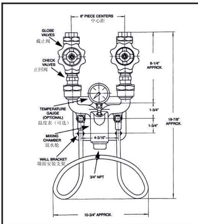
正视图
