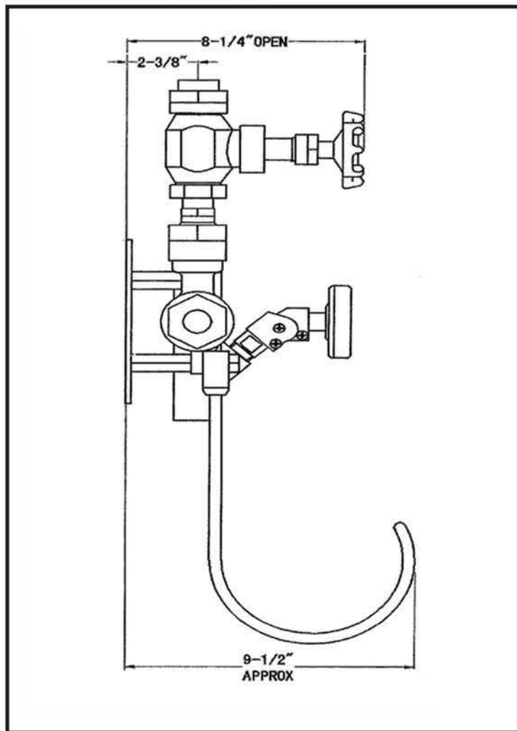
侧视图
