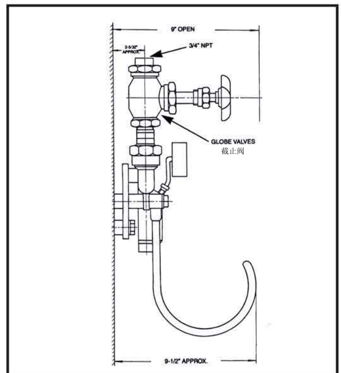
侧视图
