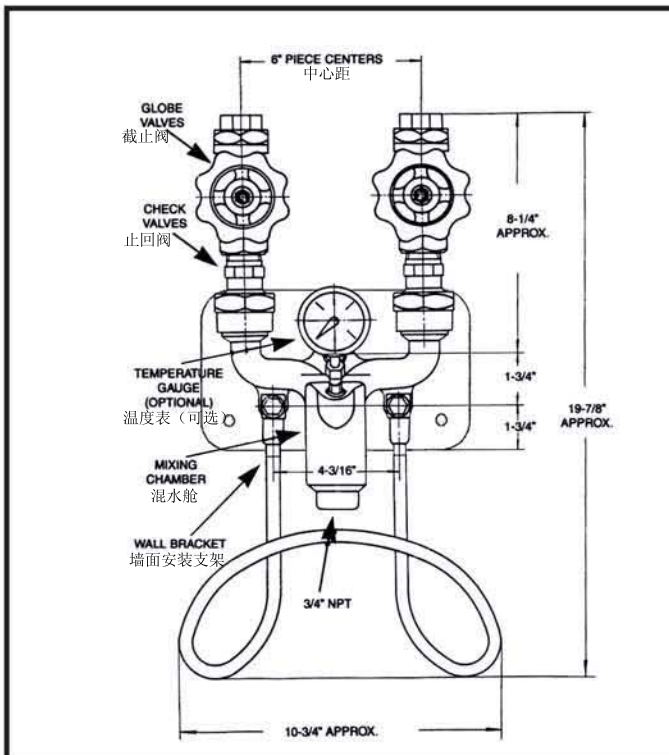
正视图
