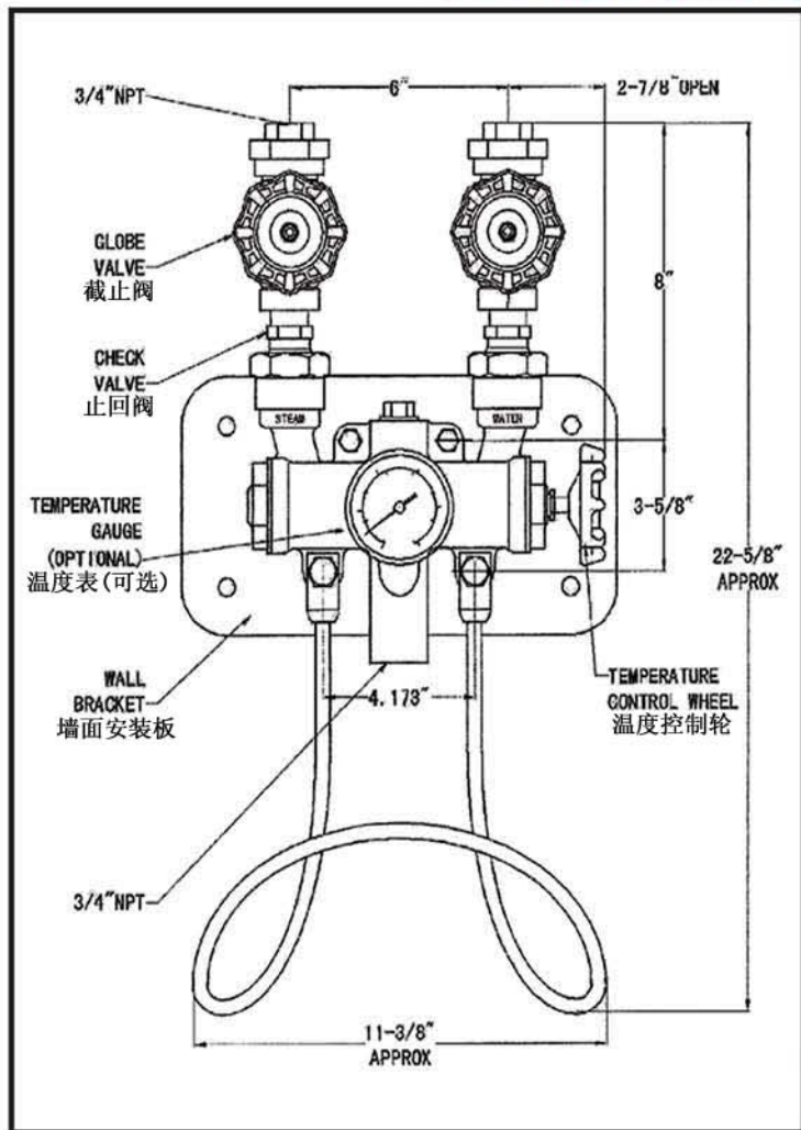
正面图
