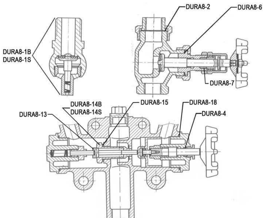
正面图
